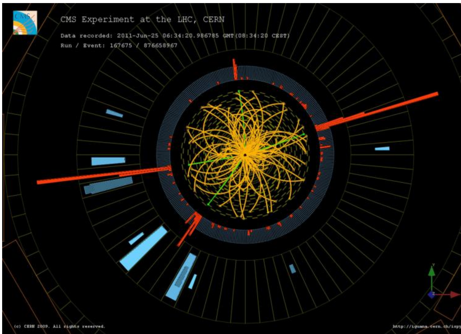
Il bosone di Higgs.
